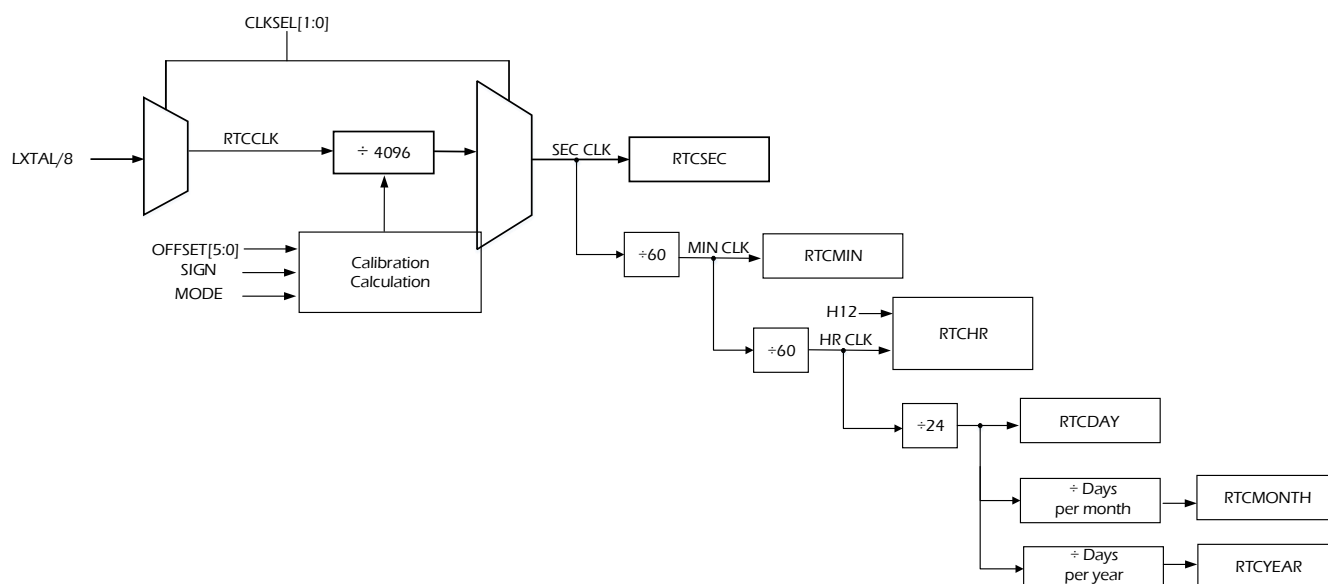
图 12-9 RTC 模块图
