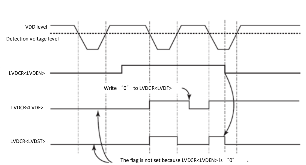
图 5-8 电压检测标帜和电压检测状态标帜的改变
