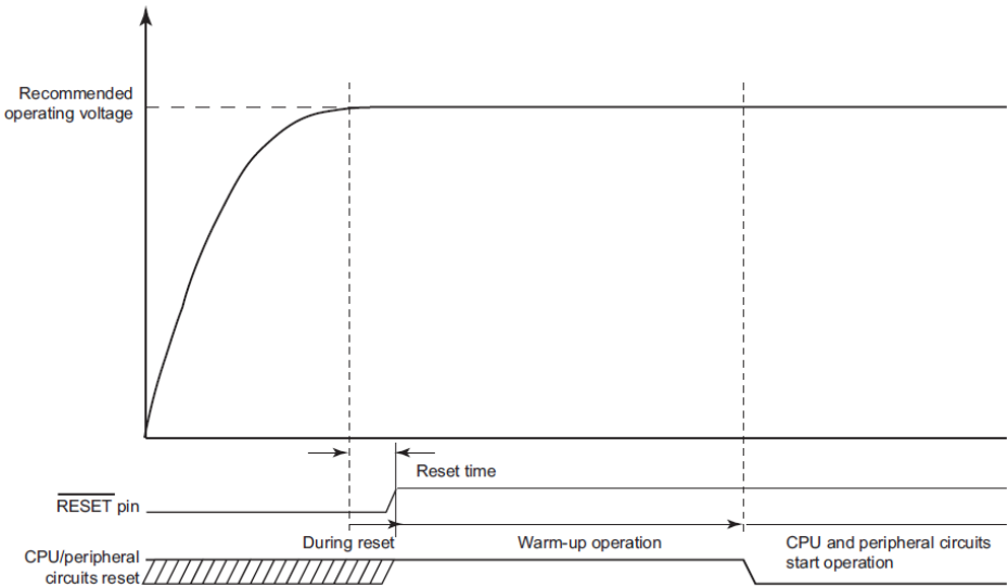
图 5-2 外部复位输入(上电时)
