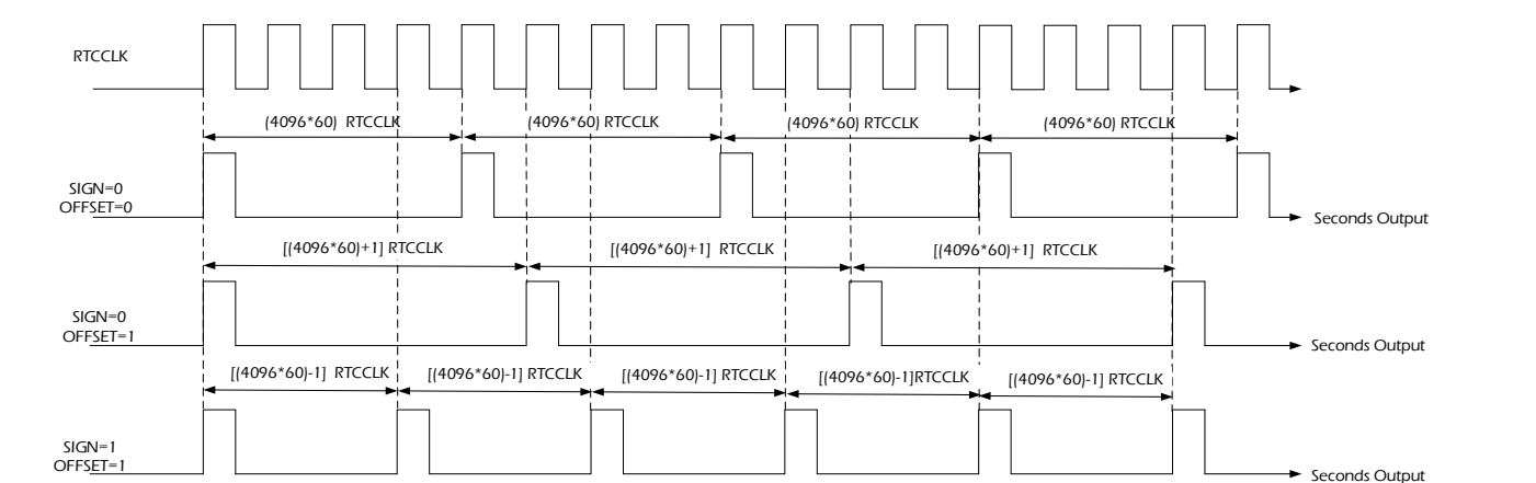
图 12-11 RTC 在 MODE=0 下校正时序范例
