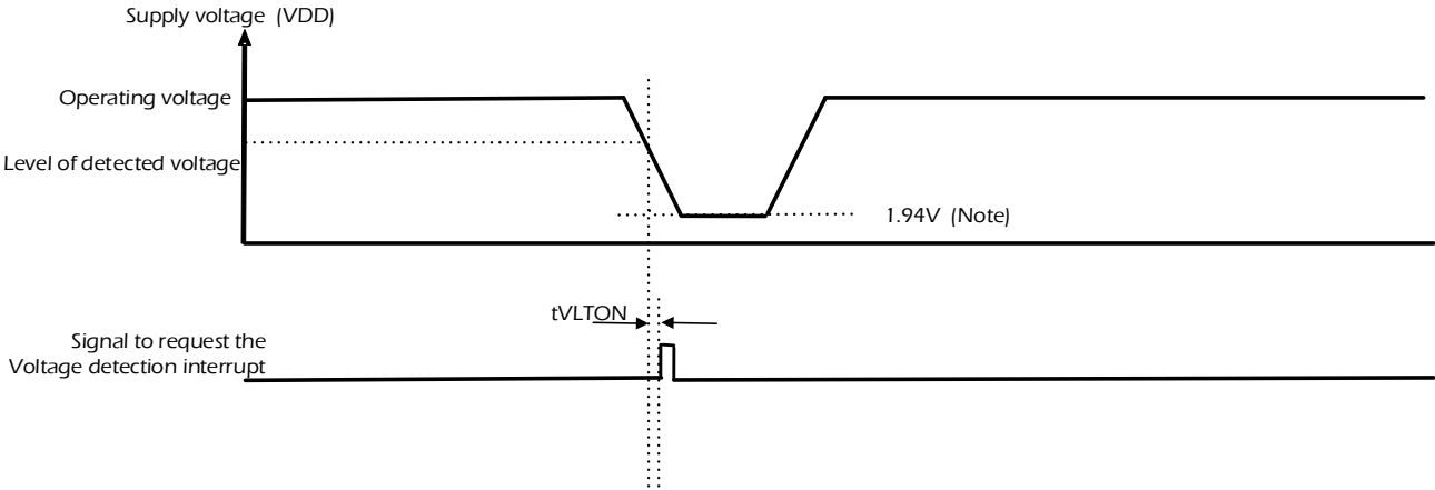
图 2- 3 LVD 中断
