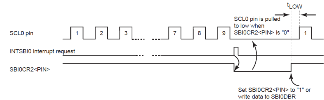
图 14- 11 SBI0CR2<PIN>与 SCL0 脚位
