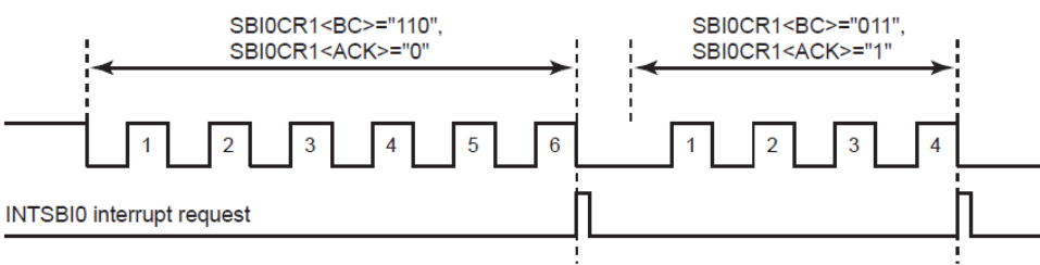
图 14- 5 数据传输时的时钟脉冲与 SBI0CR1<BC>, SBI0CR1<ACK>(图以 SBI0 作为范例)
