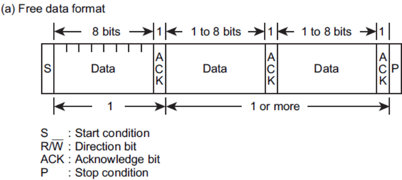
图 14- 3 通用数据模式
