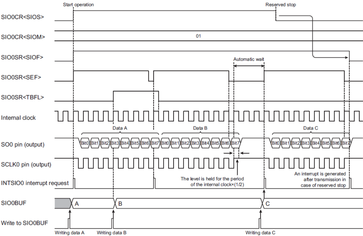
图 15-38 位元传送模式(内部时钟且预定停止)
