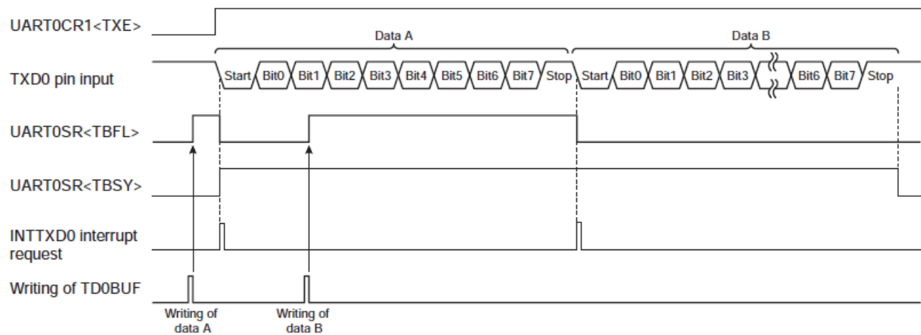
图 13- 15 发送缓存器已满的发生
