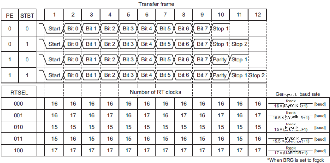
图 13-4 以 UART0CR2<RTSEL>微调波特率
