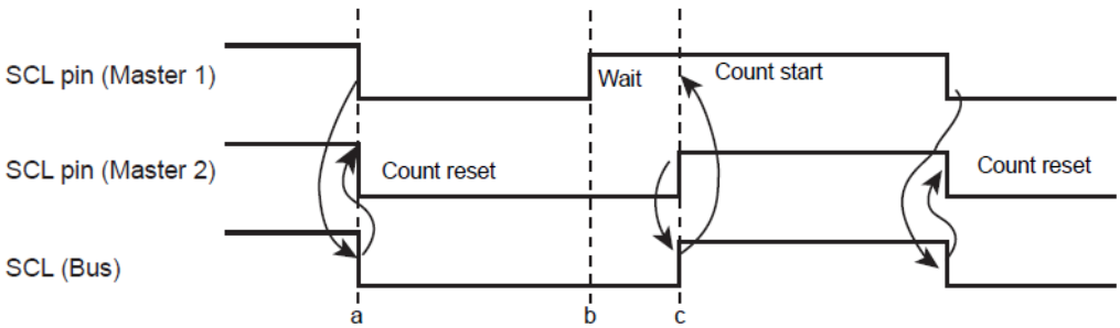
图 14- 8 同步时钟范例
