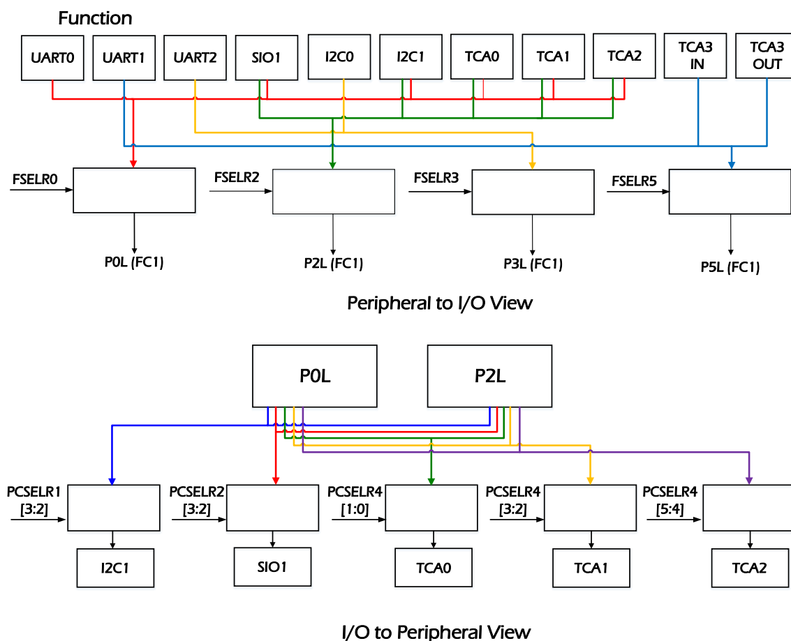
图 11-2 PNIC 架构图
