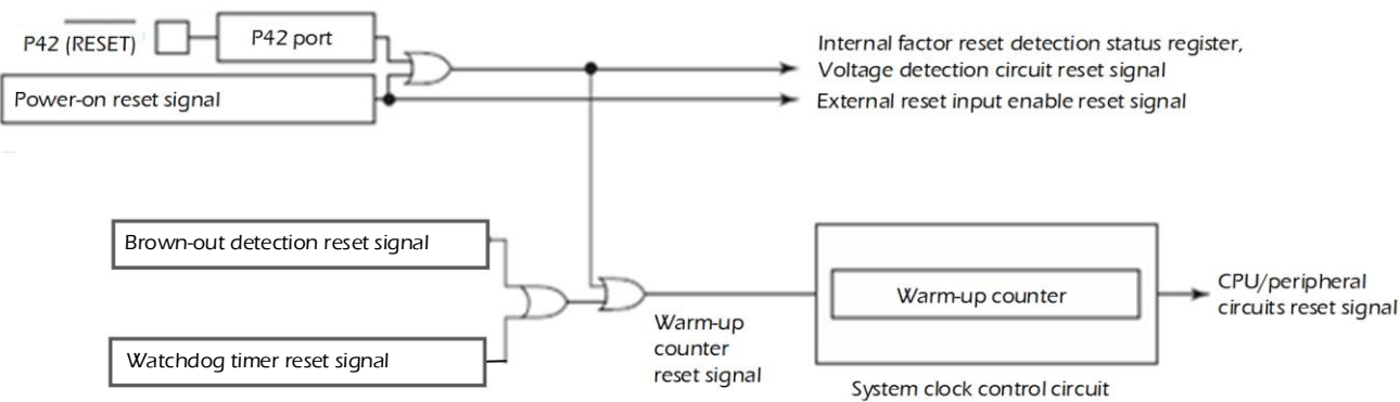
图 5- 1 复位架构
