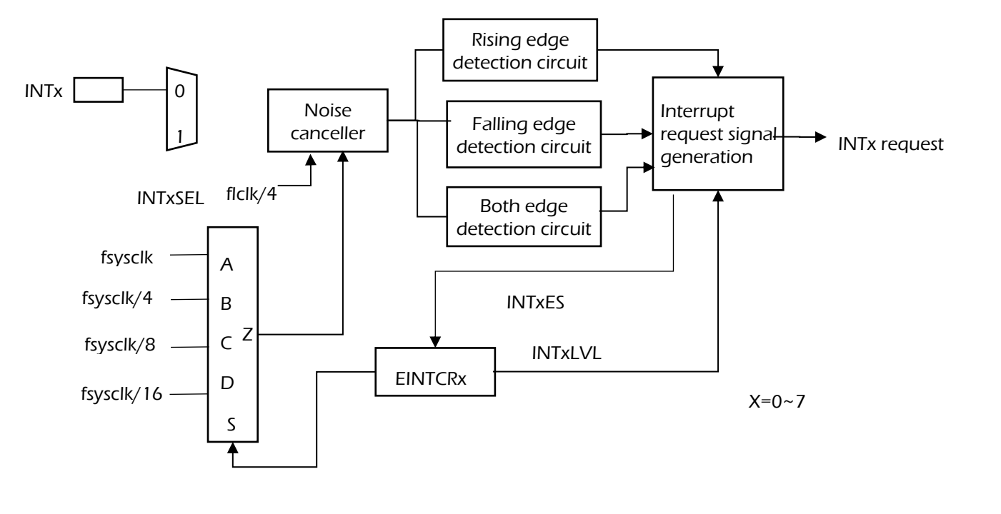
图 5-10 外部中断 (INT0~INT7)
