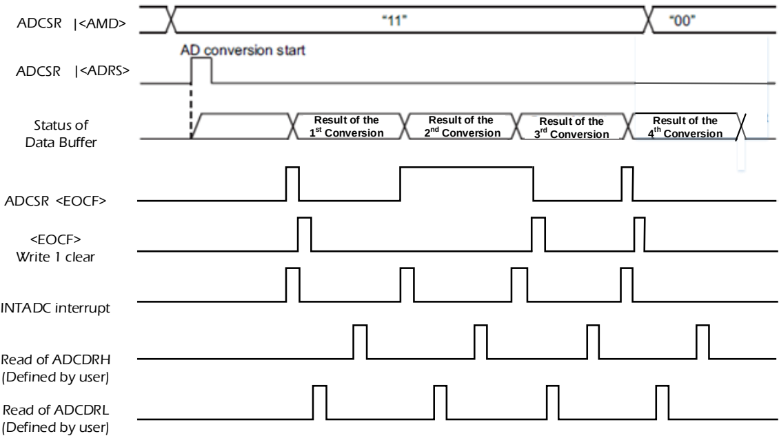
图 7- 5 ADC 重复模式
