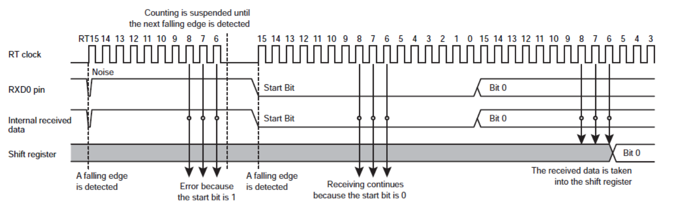
图 13-6 启始位的取样
