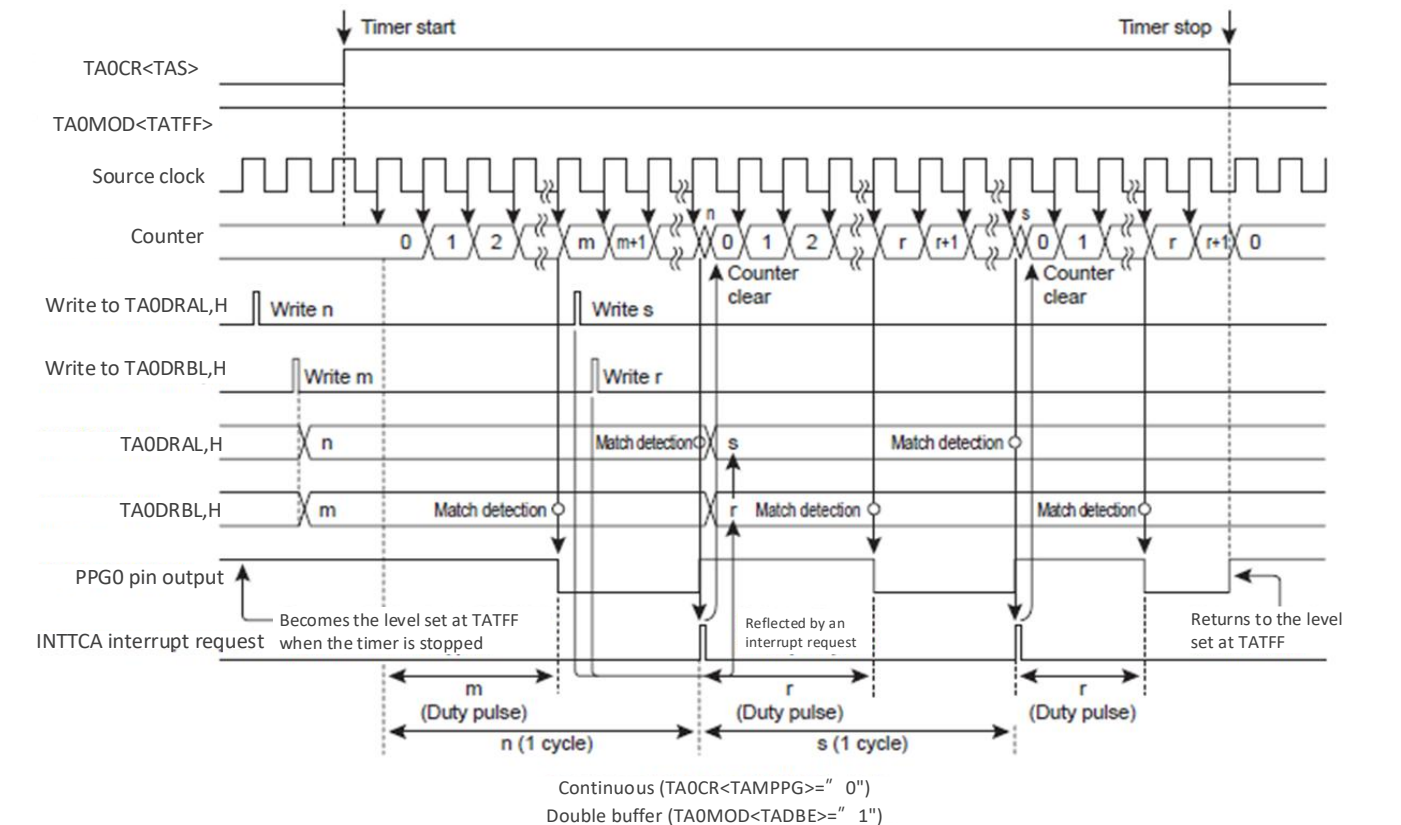
图 12- 21 PPG 模式时序图- 连续输出(TCA0 为范例)
