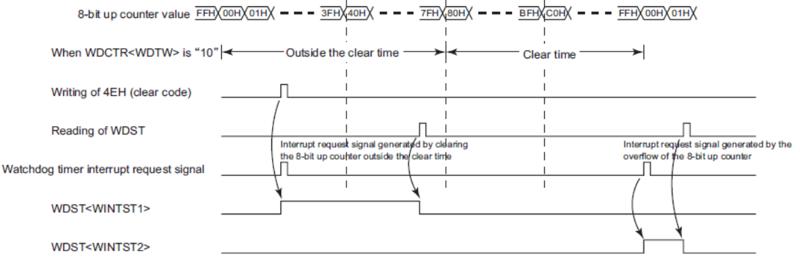
图 12-4 看门狗定时器状态
