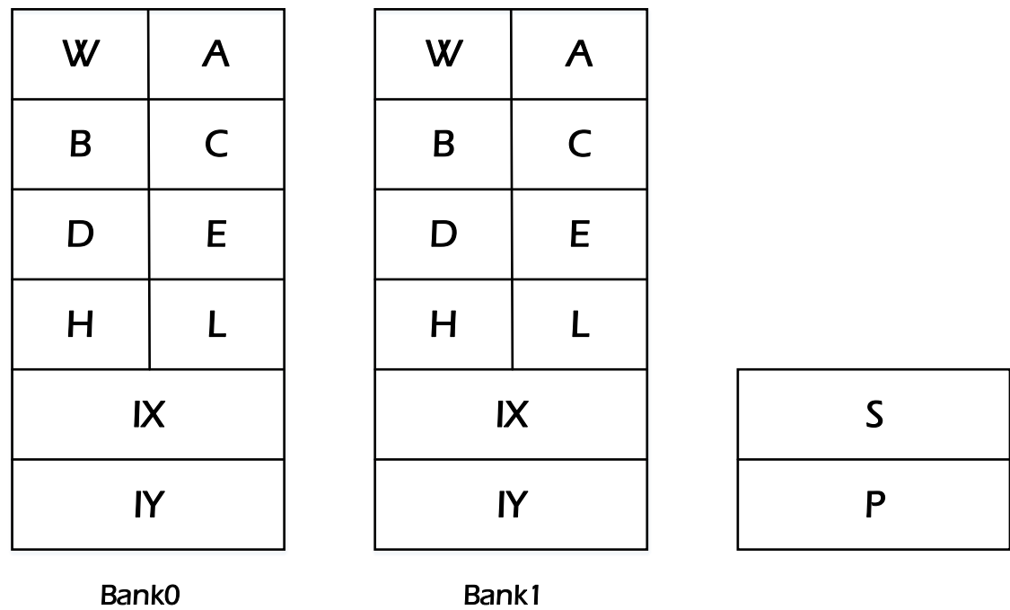
图 3-1 核心寄存器
