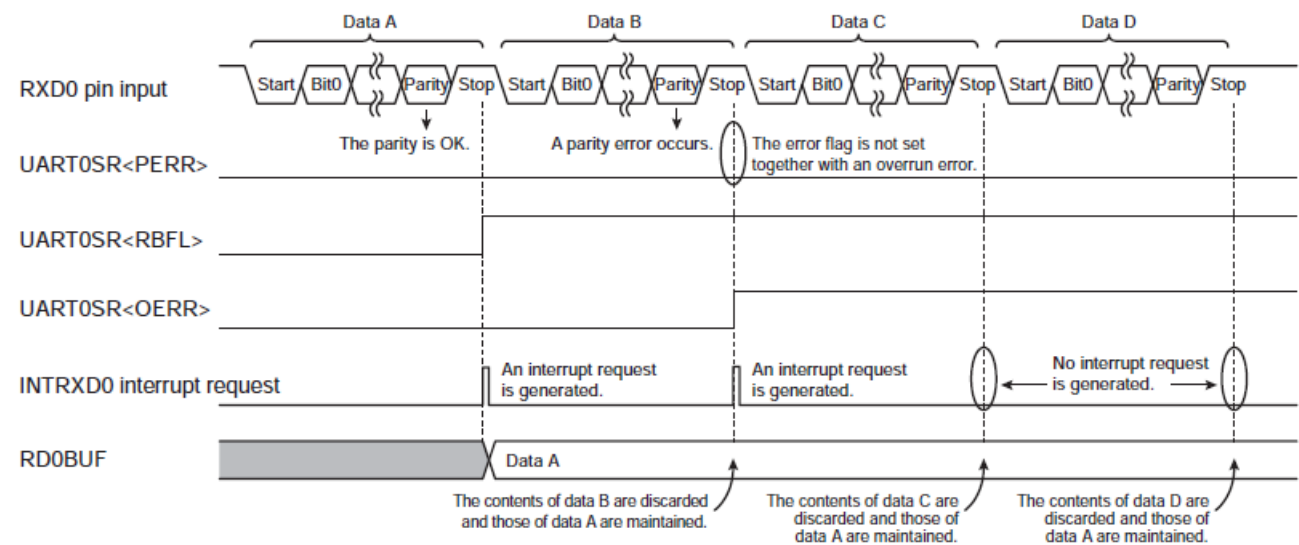
图 13- 11 发生溢出错误时的数据框/同位错误标帜
