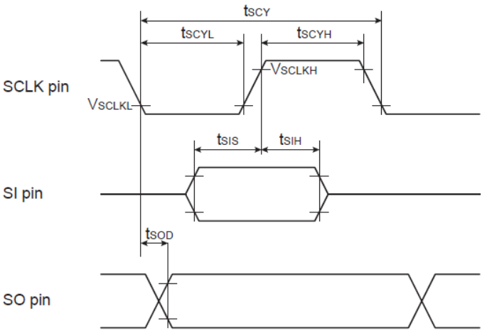
图 15- 16 AC 特性图
