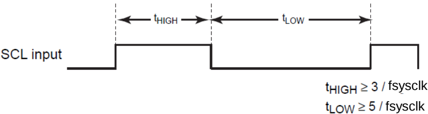
图 14- 7 SCL 输入
