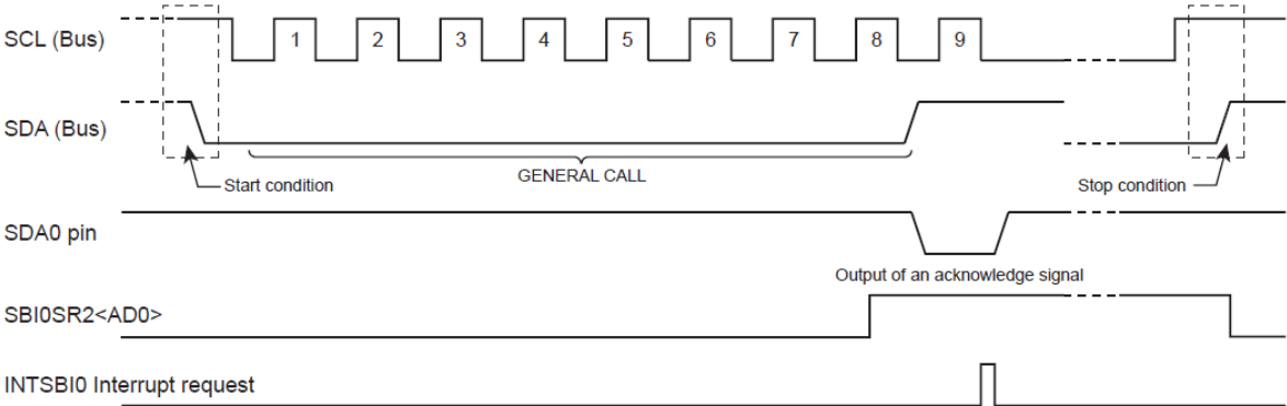
图 14- 15 广播呼叫变更(以 SBI0 为范例)
