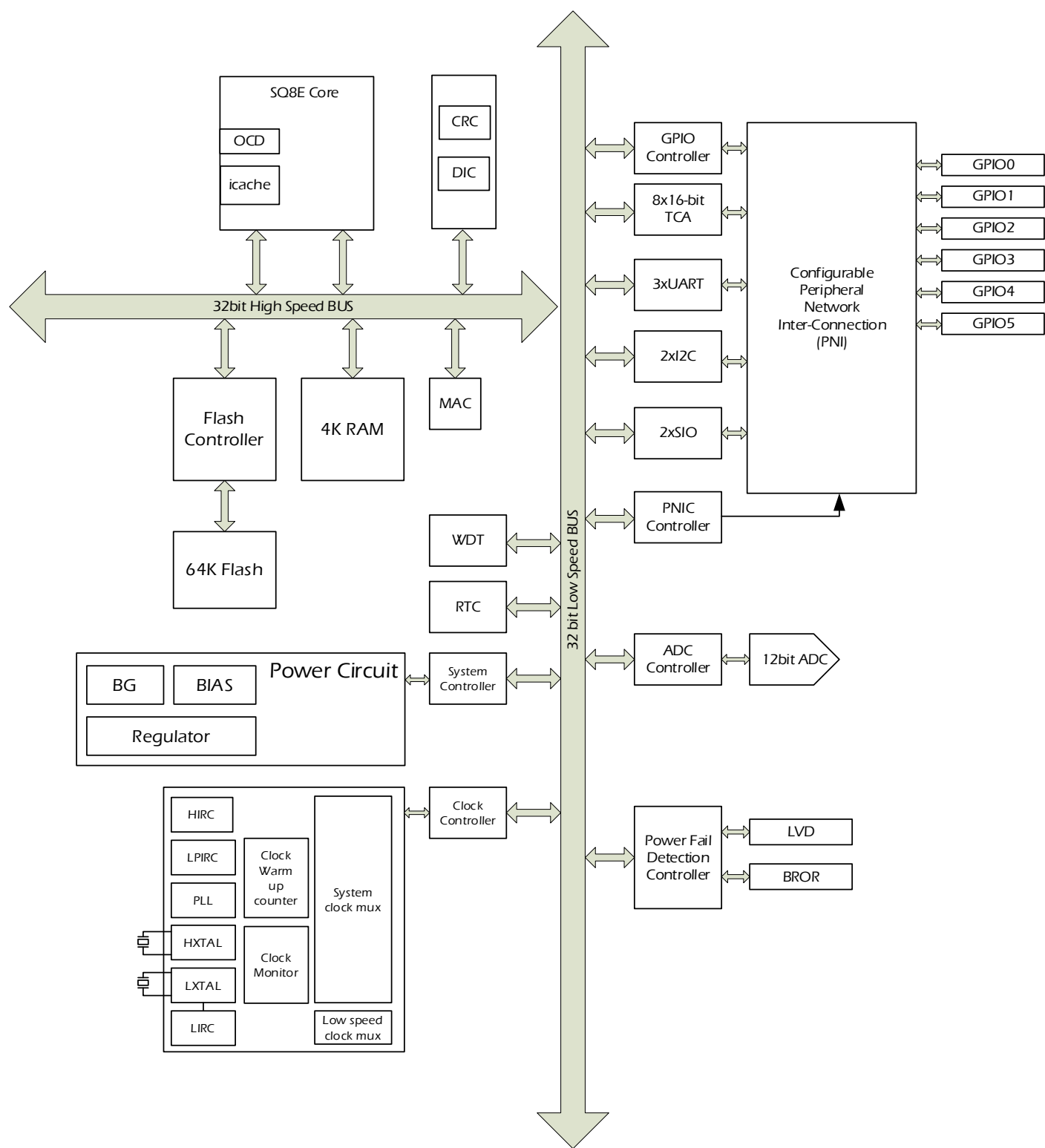
图 1-2 系统模块图
