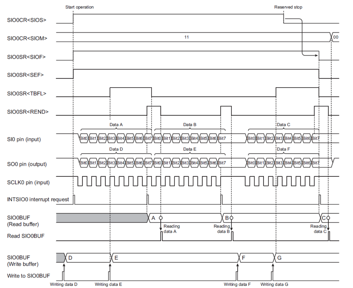
图 15- 148 位发送/接收模式(外部时钟且预约停止)
