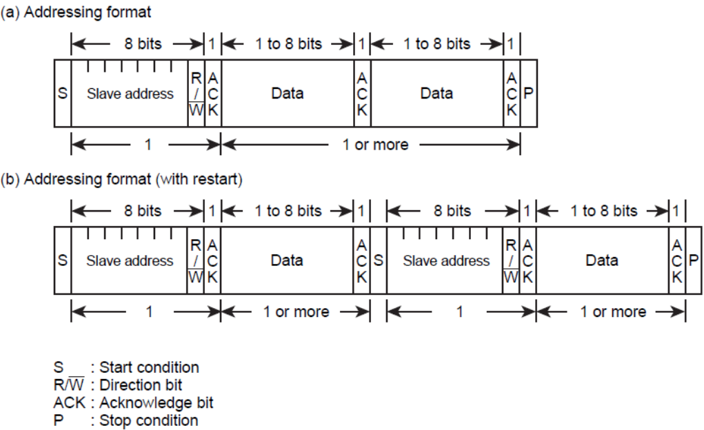
图 14- 2 I2C 总线数据格式
