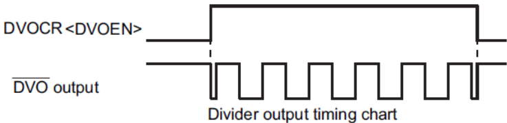
图 12- 6 分频器输出时序
