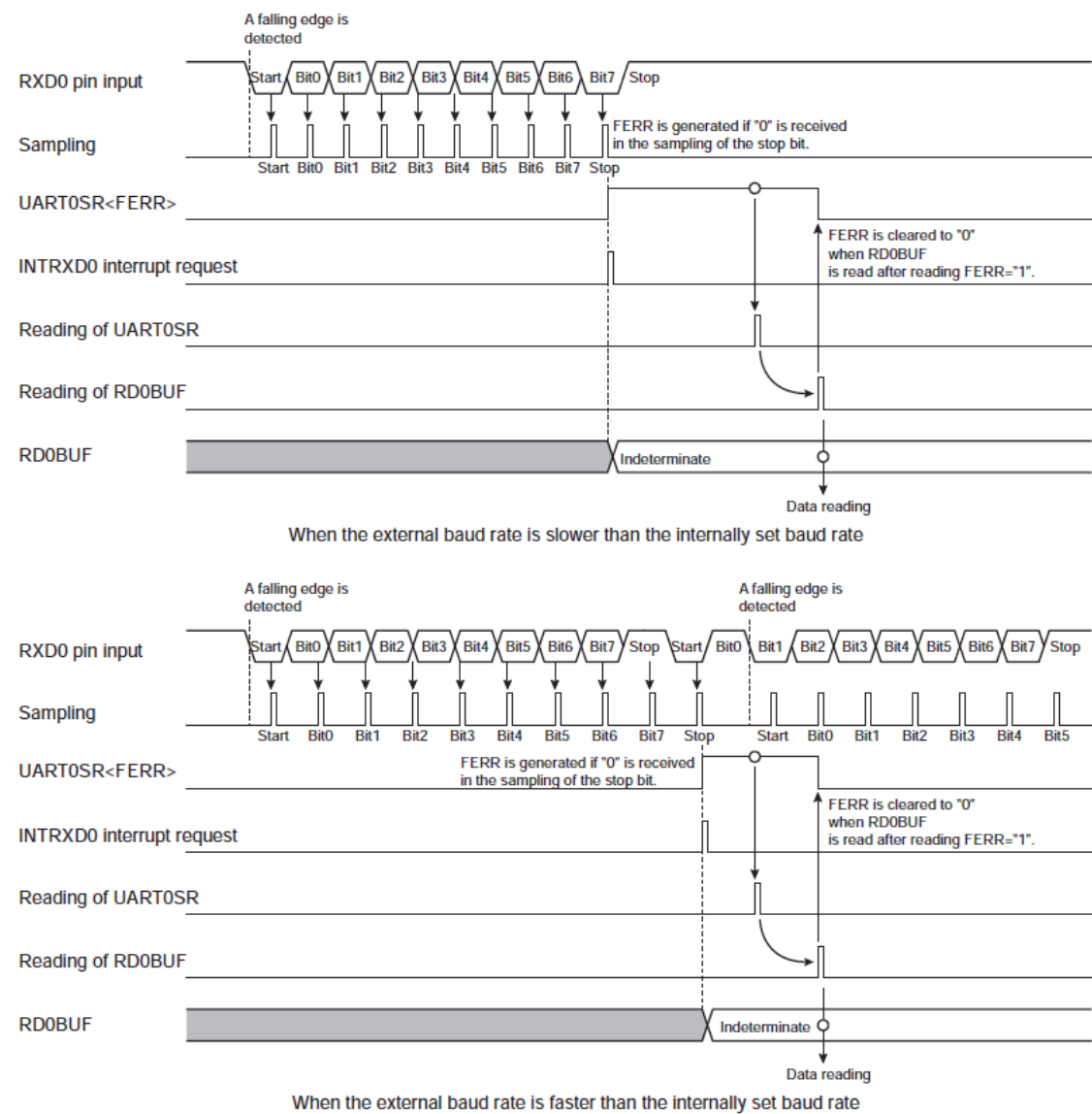
图 13-9 数据框错误的发生
