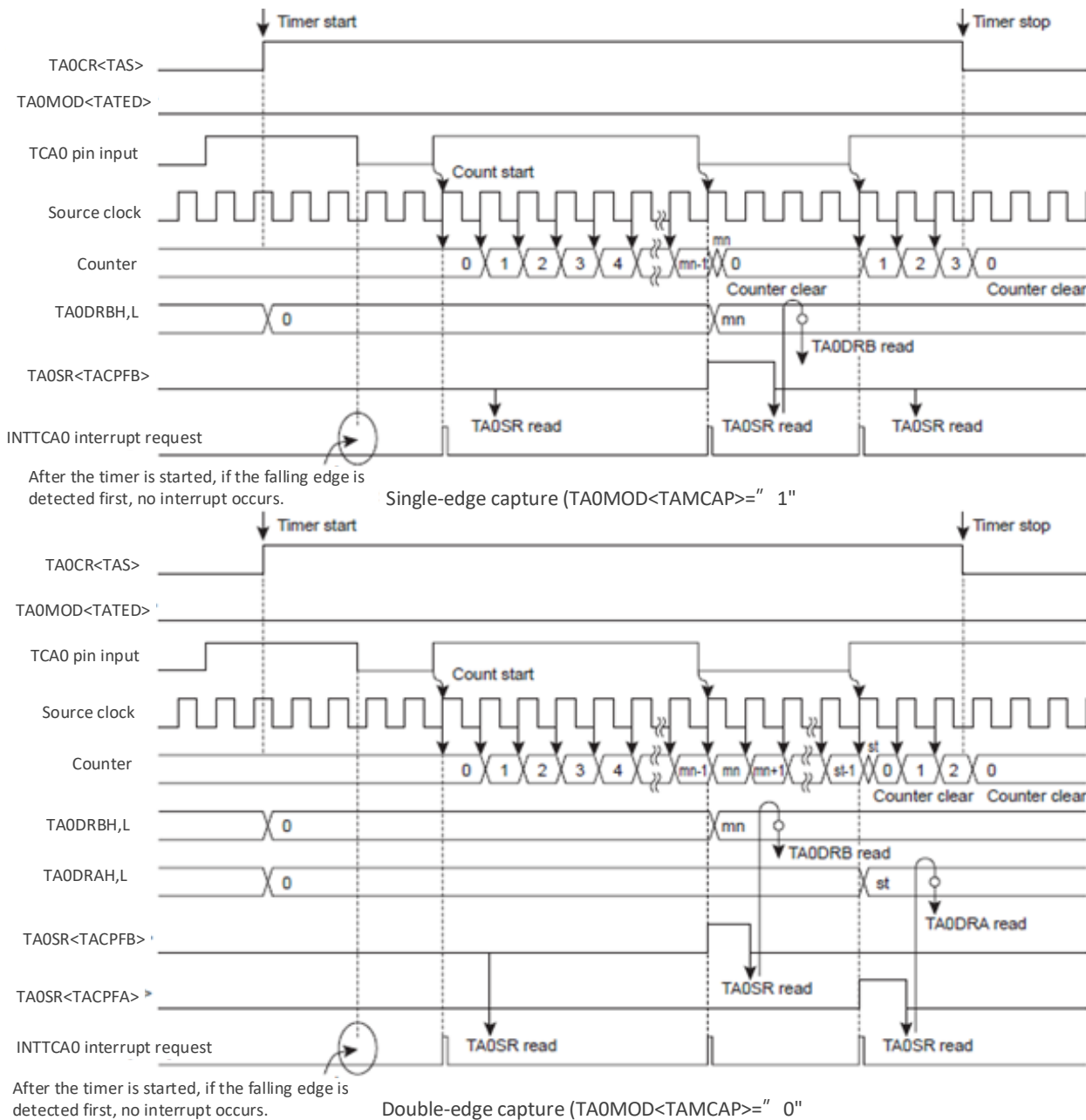
图 12- 18 脉宽测量模式时序图(TCA0 为范例)
