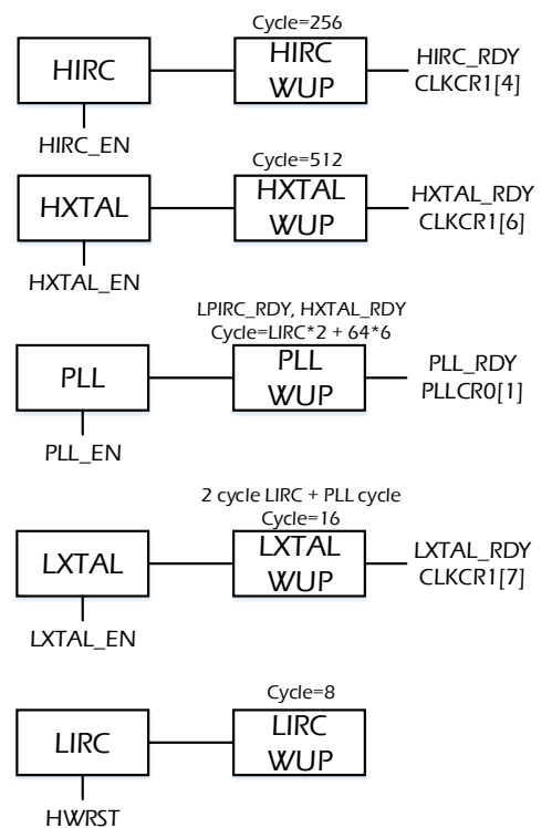
图 6-2 各时钟启动行程及所需周期
