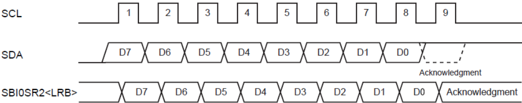
图 14- 16 最后接收位变更监控(以 SBI0 为范例)
