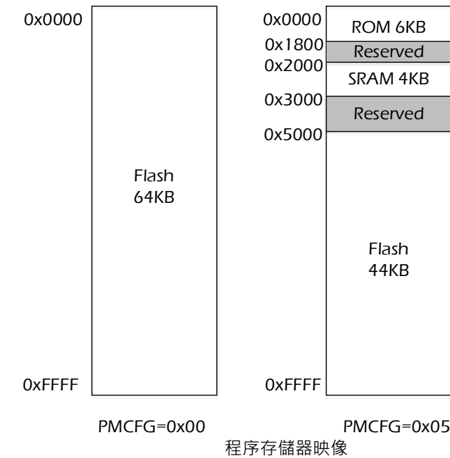
图 4-1 程序存储器映像
