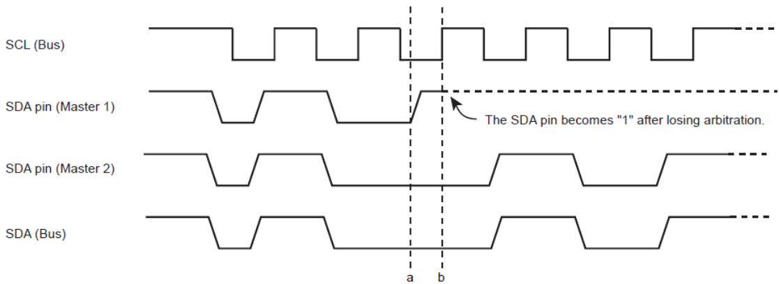
图 14- 12 仲裁丢失
