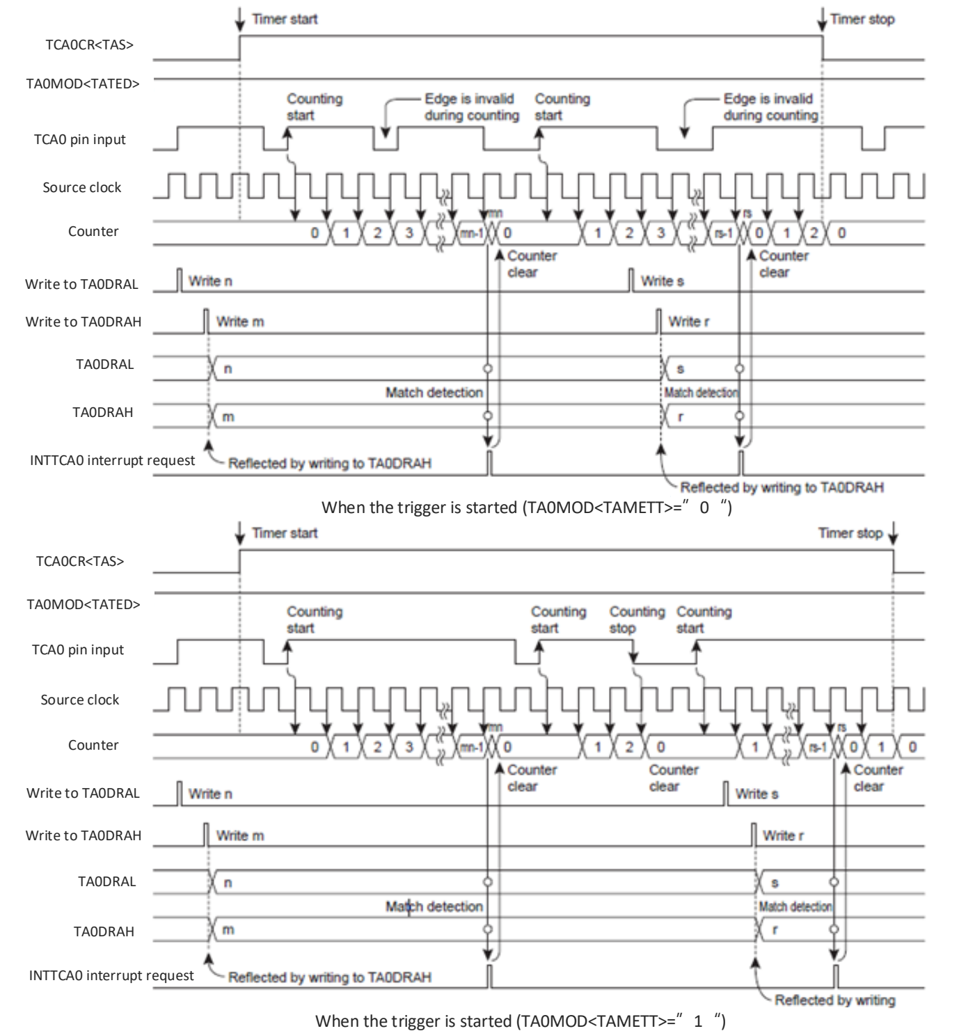
图 12- 15 外部触发定时器模式时序图(TCA0 为范例)
