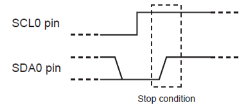
图 14- 10 停止条件产生(以 SBI0 为例)
