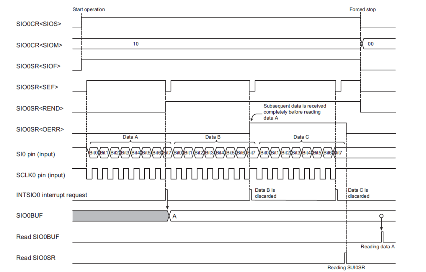
图 15- 12 8 位接收模式(外部时钟与溢出错误发生)
