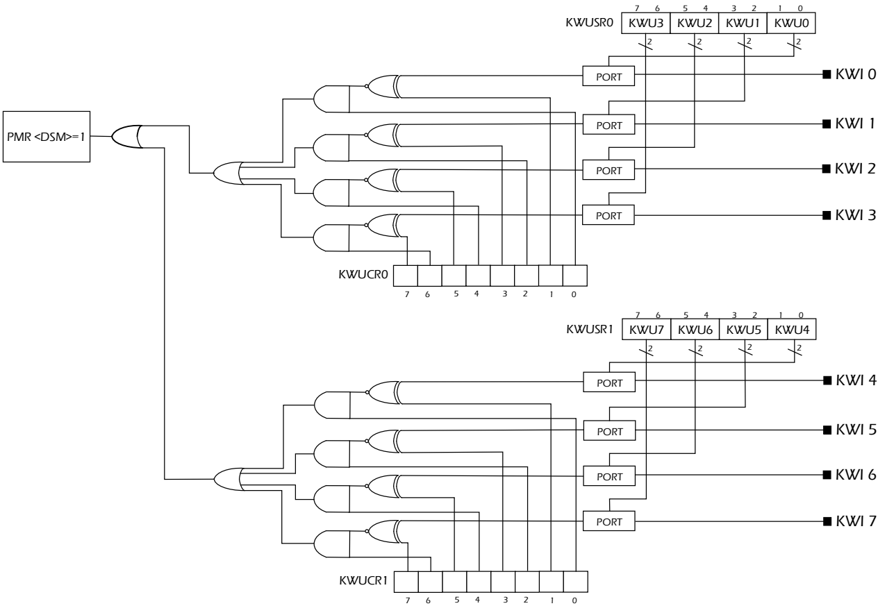
图 5-9 唤醒线路(以 KWIO~ KWI7 为例)
