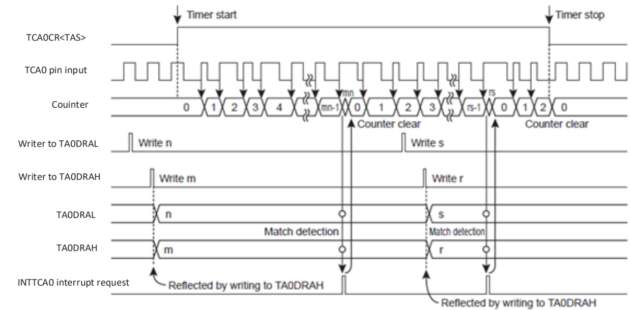
图 12- 16 事件计数器模式时序图(TCA0 为范例)
