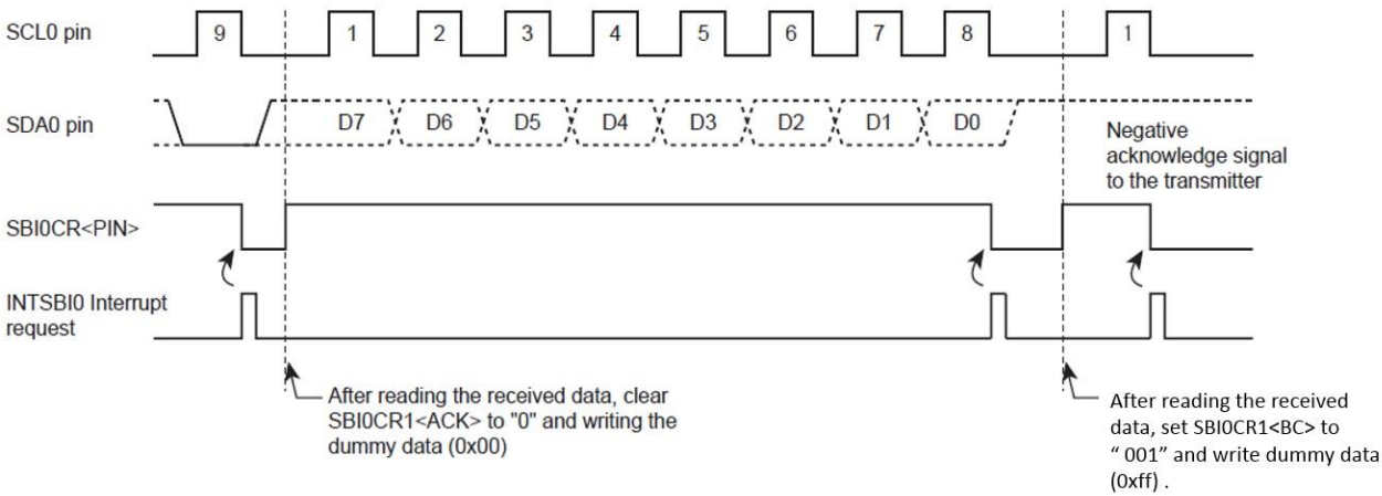
图 14- 20 在主机接收模式下的数据传输中止(以 SBI0 为例)
