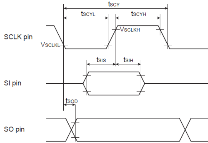
图 15.16 AC 特性
