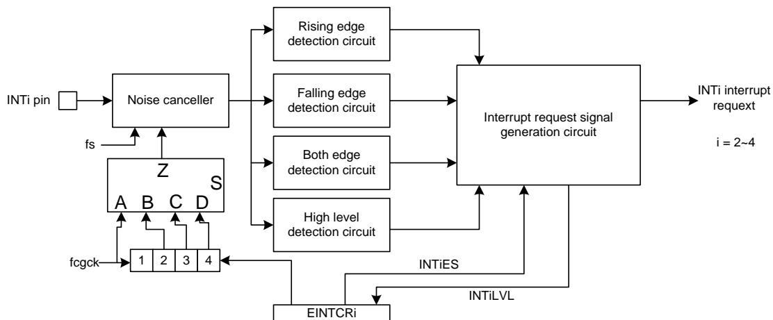
图 7.2 外部中断 2/3/4
