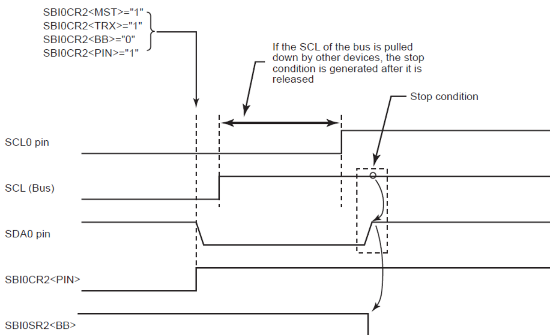
图 14.21 停止条件产生
