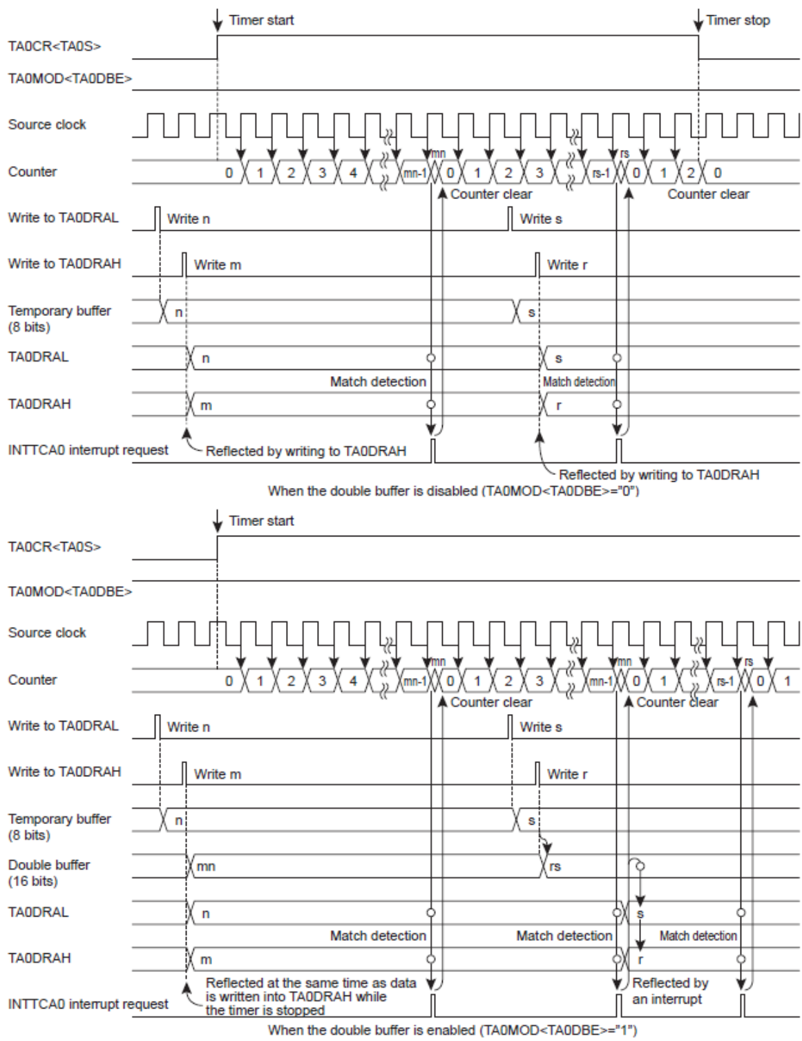
图 10.49 定时器模式时序图
