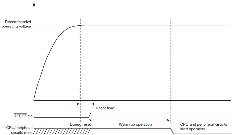
图 5.2 外部复位输入(上电时)
