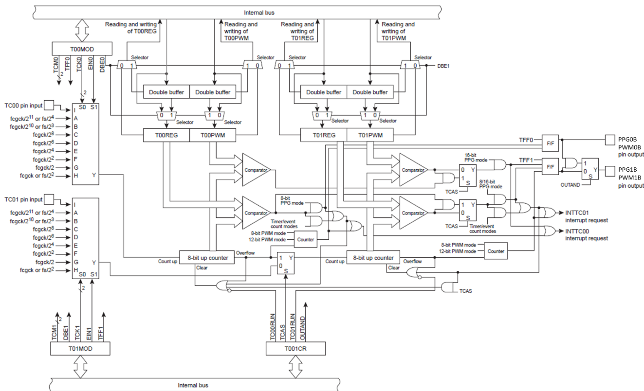
图 10.10 8 位定时器计数器
