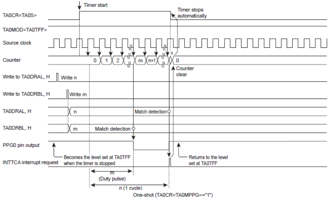
图 10.56 PPG 模式时序图- 单次输出
