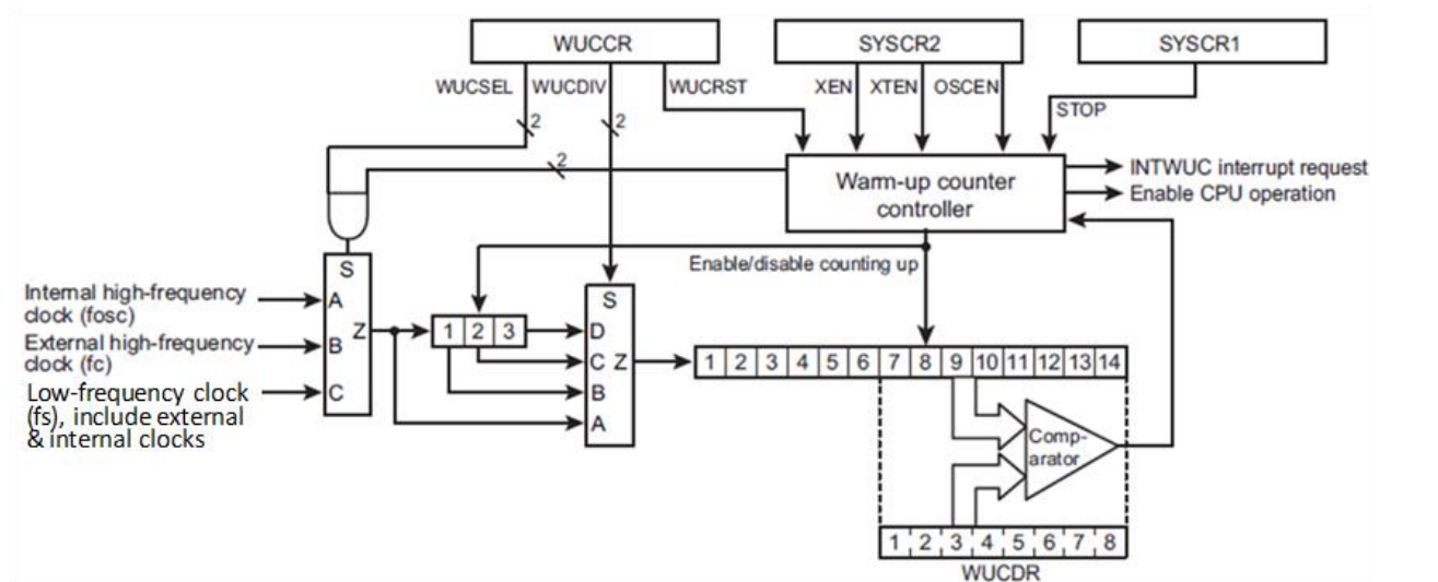
图 6.4 唤醒计数器线路
